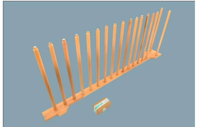
2. Voeg de sporten toe in 1 zijde van de 1 van de 2 zijpanelen
