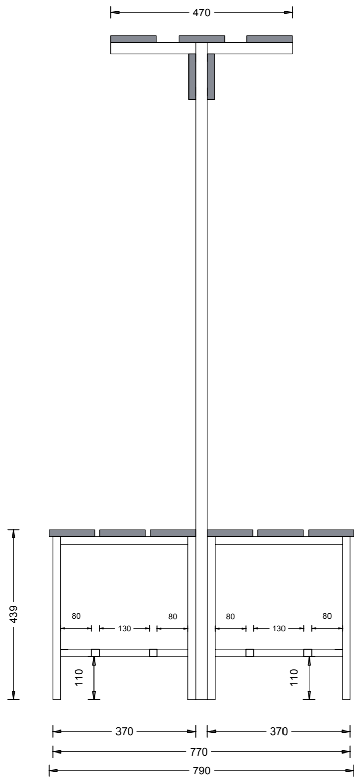
SECTIUNE TRANSVERSALA SC. 1 :10
