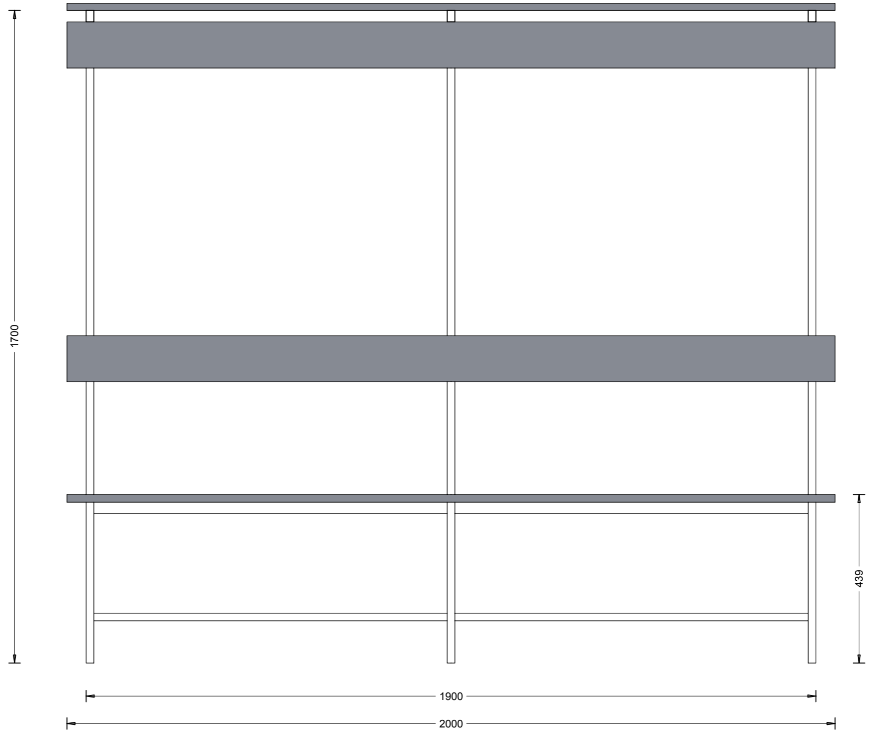
VEDERE FRONTALA SC. 1 :10
